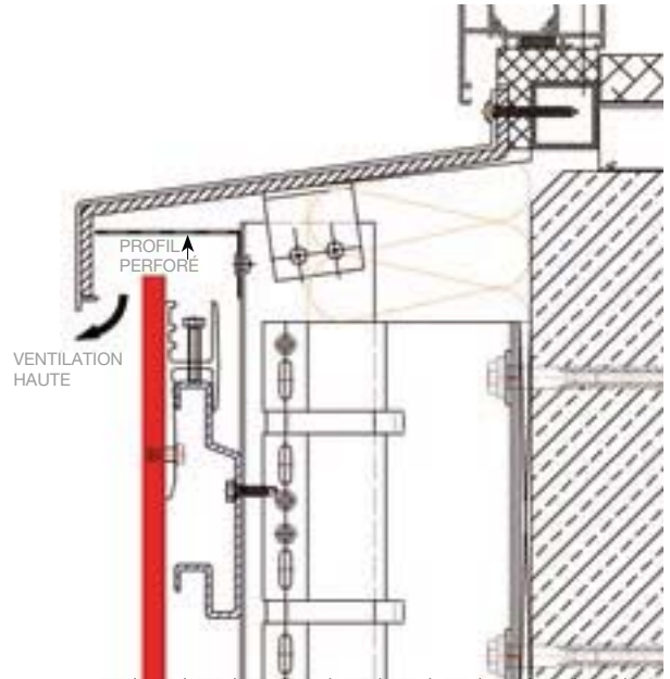
DÉTAIL APPUI DE FENÊTRE
