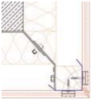
ANGLE SORTANT SANS PROFILÉ
