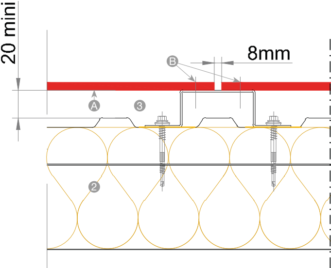
SECTION COURANTE
