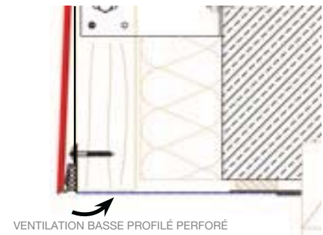
DÉTAIL LINTEAU
