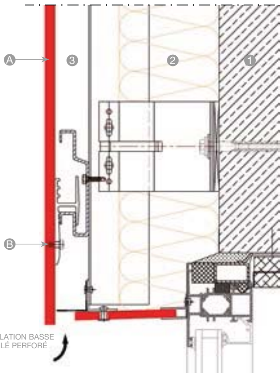
DÉTAIL LINTEAU
