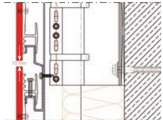
DÉTAIL JOINT HORIZONTAL
