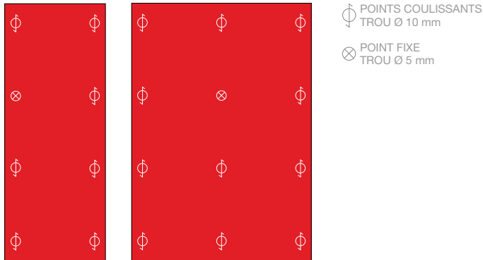
POSE SUR 2 APPUIS
