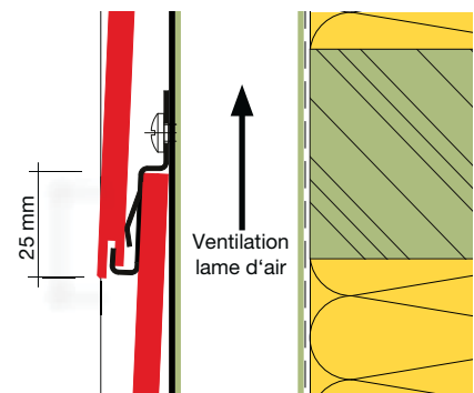
RECouvrement DES PANNEAUX SCALEO
