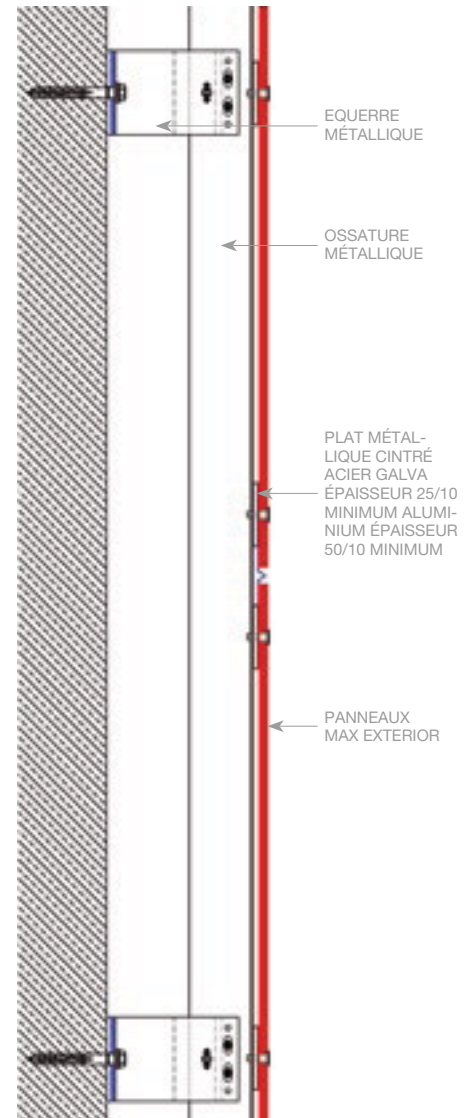
COUPE VERTICALE
