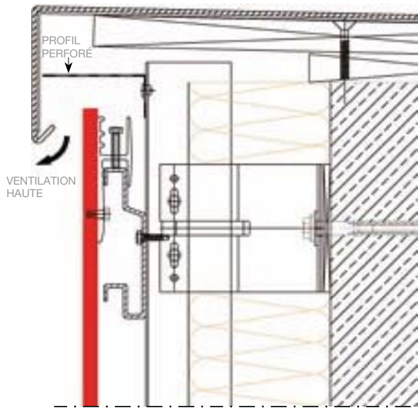
DÉTAIL COUVERTINE
