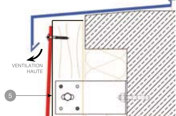
DÉTAIL APPUI DE FENÊTRE
