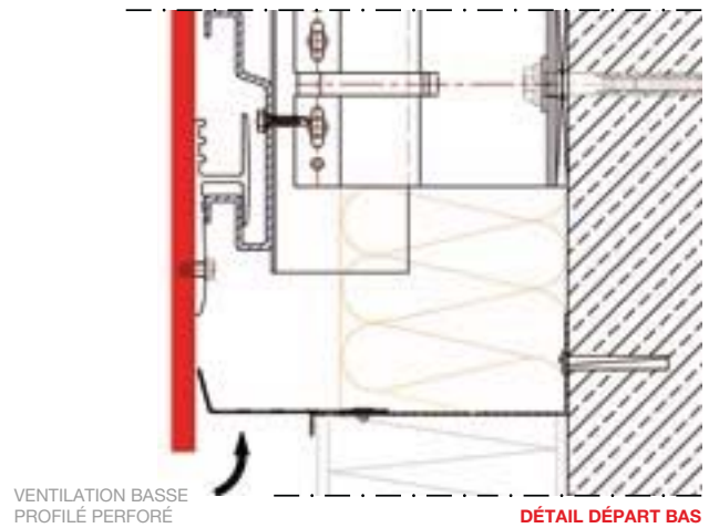
DÉTAIL DÉPART BAS
