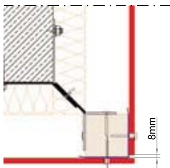
ANGLE SORTANT
