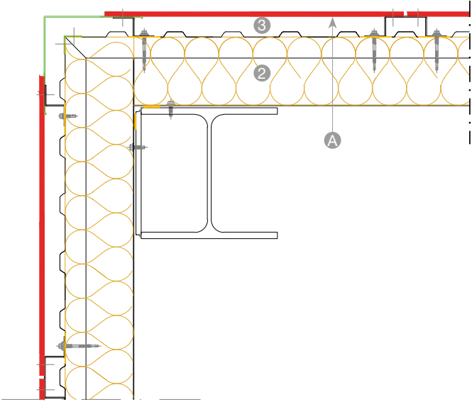
DÉTAILS D'ANGLE
